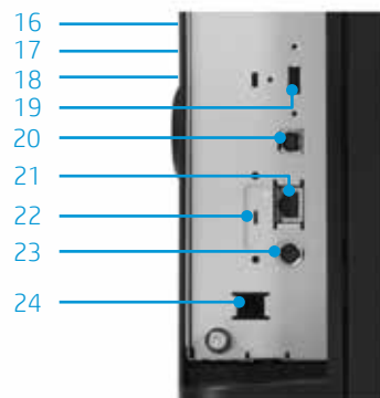
Immagine dettagliata del pannello I/O laterale
