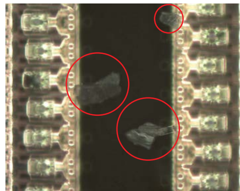
As partículas de tintas de outros fabricantes entopem os canais de tinta das cabeças de impressão, causando falha nos bocais, faixas e falha nas cabeças de impressão
