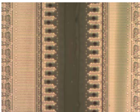
Canais de tinta das cabeças de impressão "limpos"
