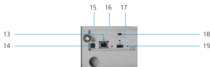
Gros plan sur le panneau d'E/S arrière
