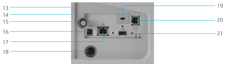
Gros plan sur le panneau d'E/S arrière
