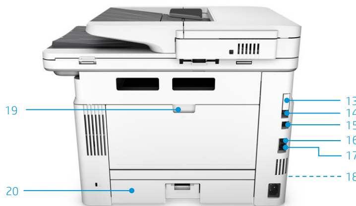
Vista posteriore
