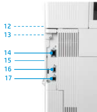
Detalhe do painel de E/S traseiro
