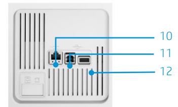
Detalle del panel de E/S posterior
