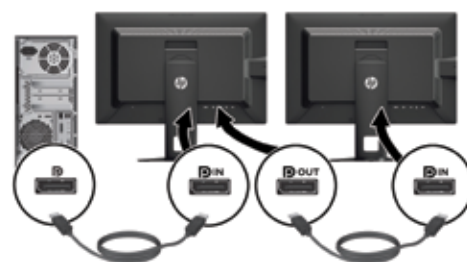
Collegamento a cascata dei display HP Z
