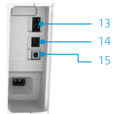
Detalle del panel de E/S posterior
