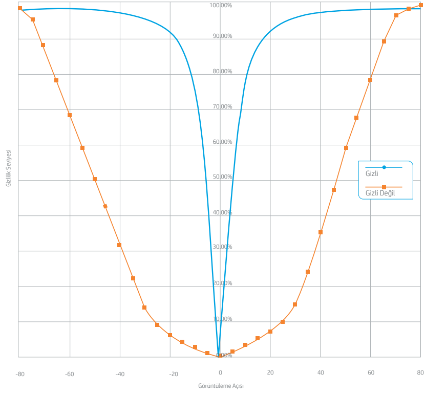
Şekil 3b. Gizli ve gizli olmayan görüntüleme bölgeleri – HP EliteBook 840 G3/G4, 1040 G3
