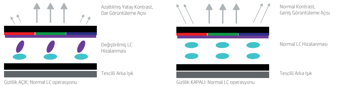
Şekil 1b. Aydınlatma operasyonu – HP EliteBook x360 1030 G2
