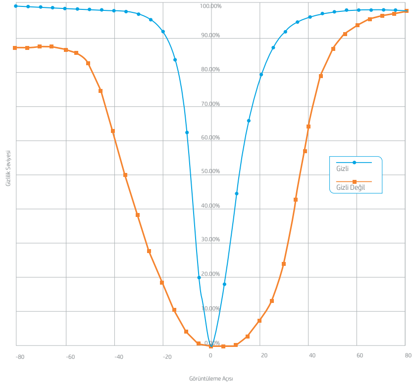
Şekil 3a. Gizli ve gizli olmayan görüntüleme bölgeleri – HP EliteBook 840 G3/G4, 1040 G3
